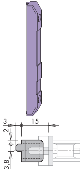
Schließblech A0213 - rechts
