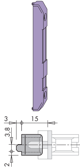
Distanzstück A0085
