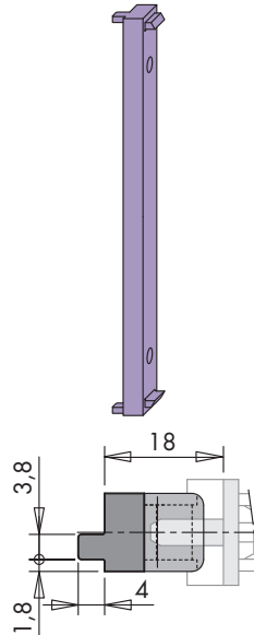
Distanzstück A0157
